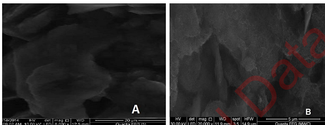
ESI 1. The SEM of CPE (A) and MWCNTCPE (B).
